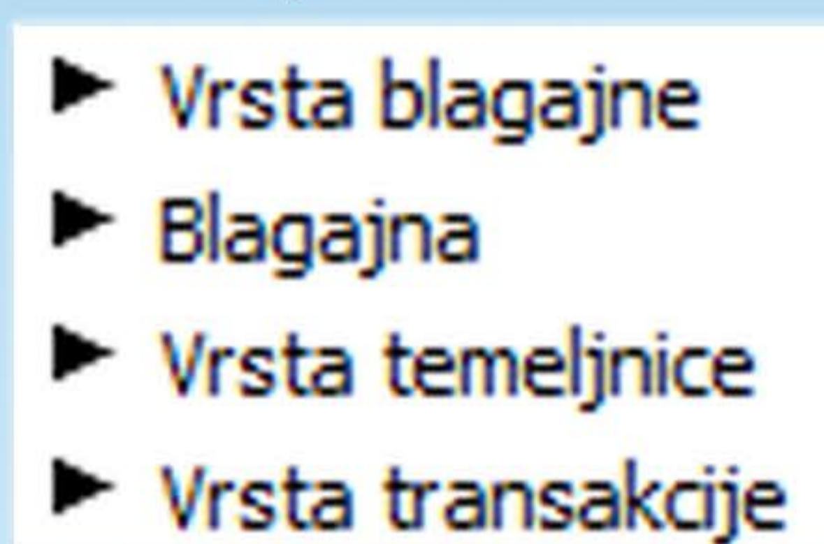
Slika: Šifarnici
